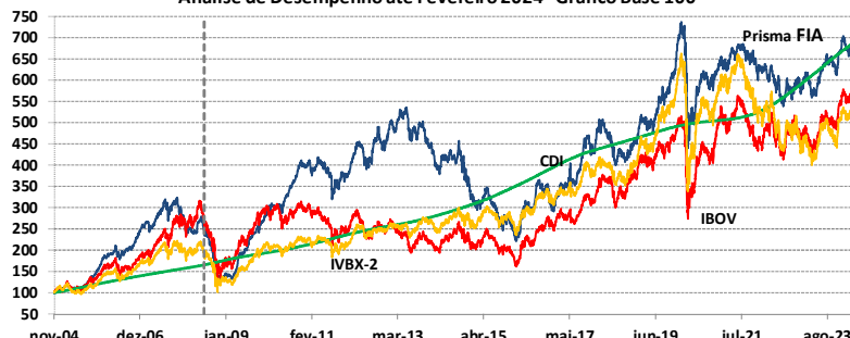
Análise de Desempenho até Fevereiro 2024 - Gráfico Base 100
