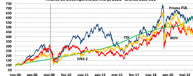
Análise de Desempenho até Março 2023 - Gráfico Base 100
